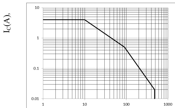
SOA
