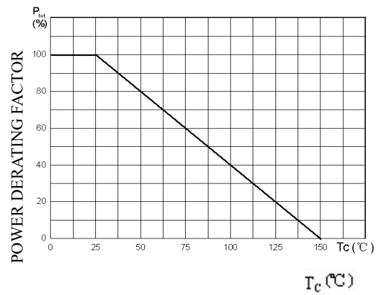
P_C - T_C
